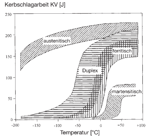
Kerbschlagzähigkeit verschiedener Edelmärkte in Abhängigkeit von der Temperatur
