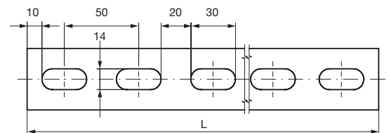
Lochbild (mm)
