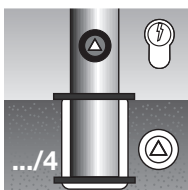
Pfeiler mit Verriegelung, herausnehmbar aus mitgelieferter Bodenhülse Poteau verrouillable, démontable à partir du socle fourni
