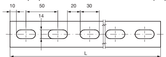
Lochbild (mm)
