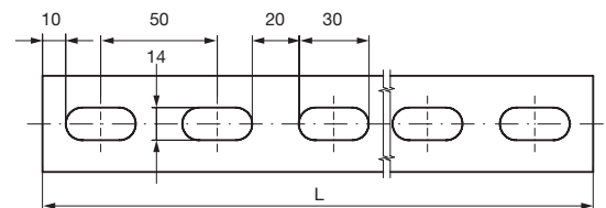
Lochbild (mm)
