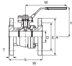
DN 15-50
