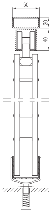
doorsnede standaard uitvoering
