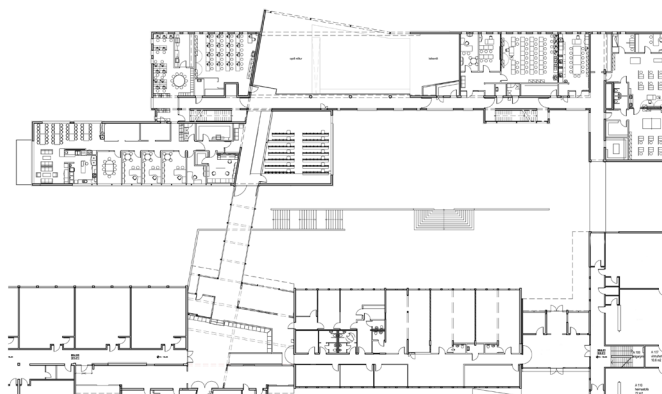
Plan 2. etg.
