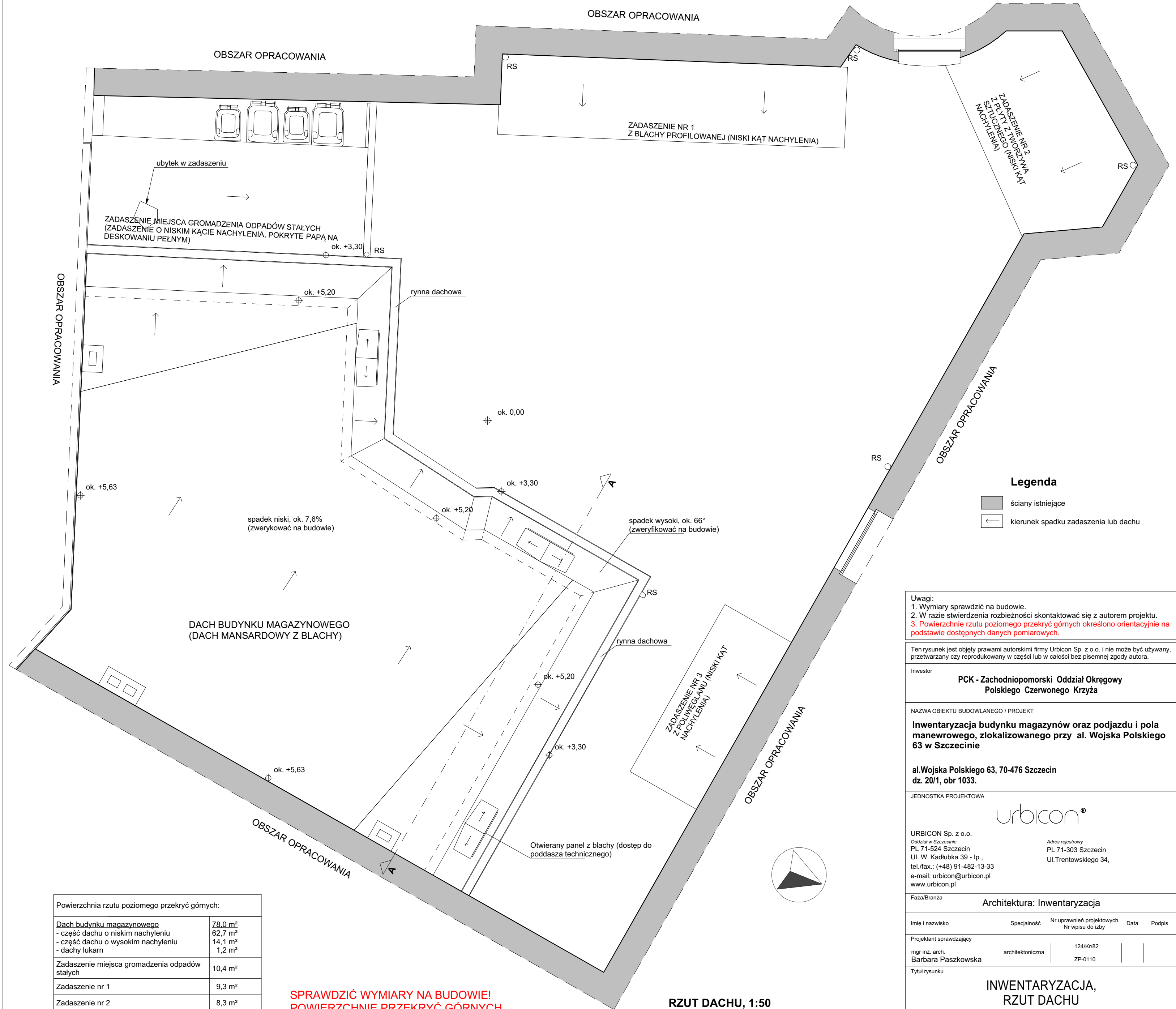
RZUT DACHU, 1:50
