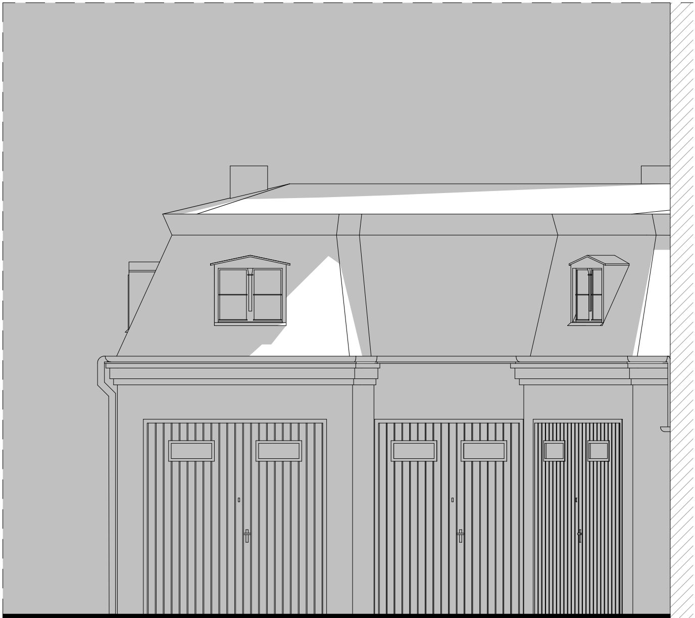
ELEWACJA ZACHODNIA, 1:50
