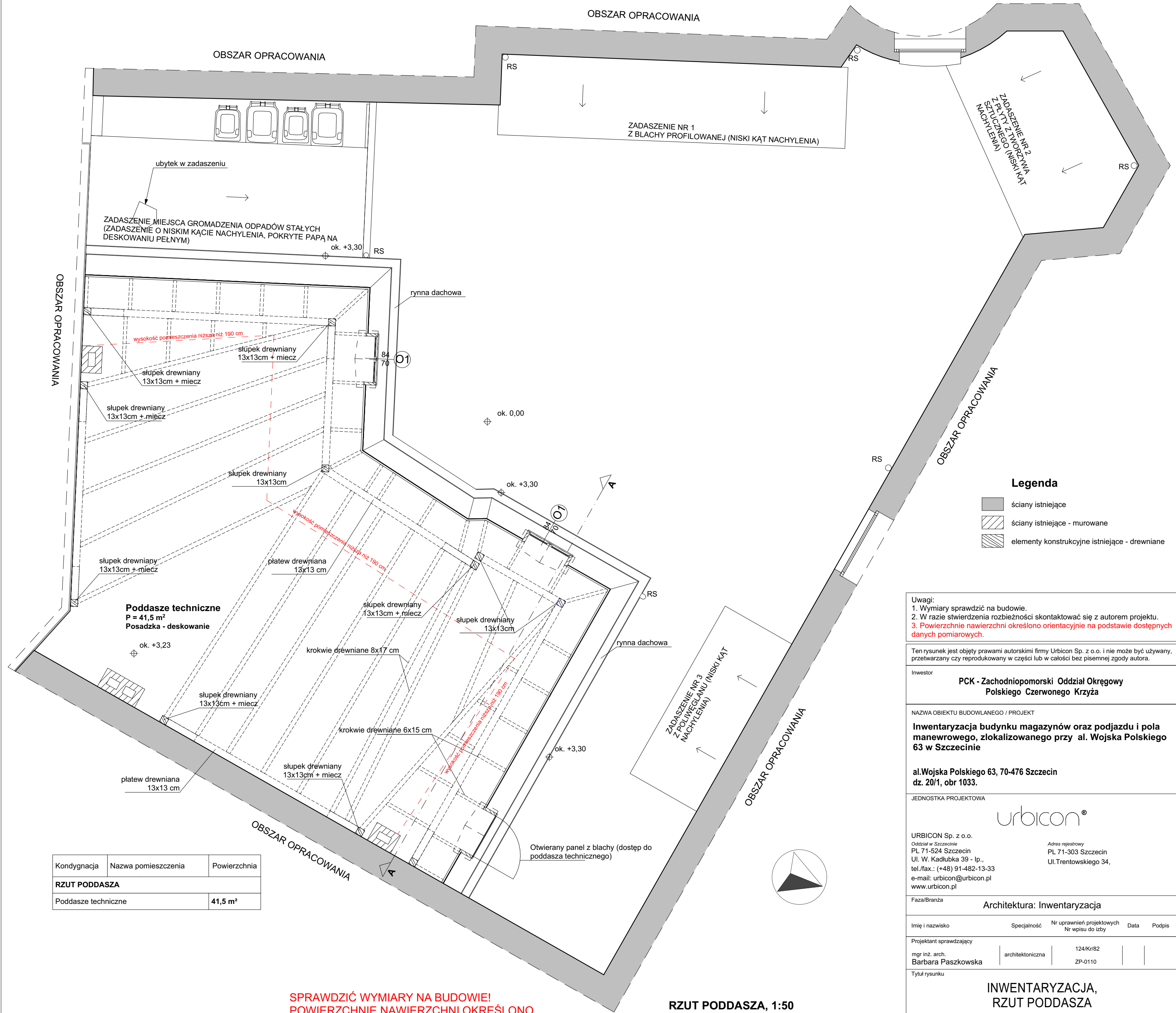
RZUT PODDASZA, 1:50
