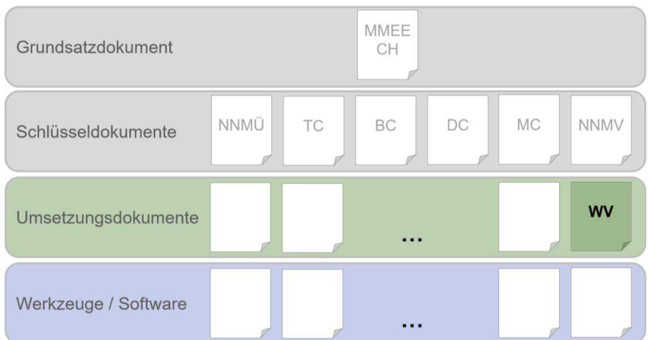
Abbildung 1: Dokumentenstruktur
