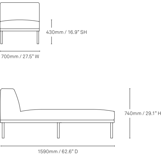
Chaise no arms
