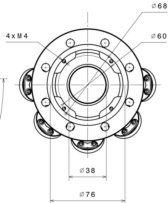
Hilfsansicht B Maßstab: 1:2
