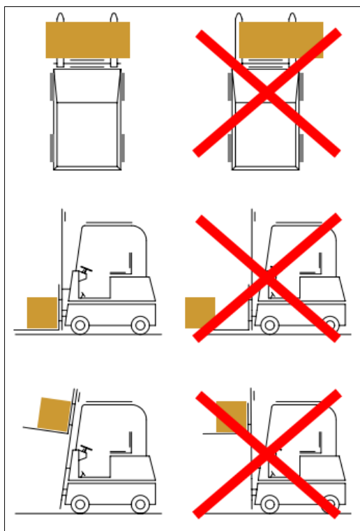
Figura 21 — Modi corretti e non corretti di utilizzo del carrello elevatore
