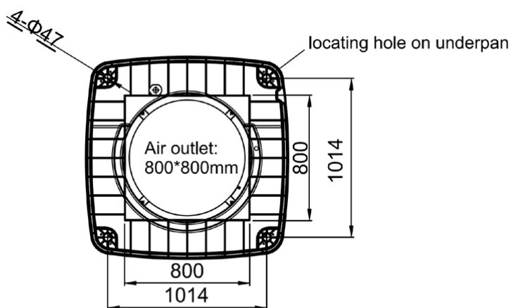
Foto 15 — Installazione raffrescatore - Vista da sotto
