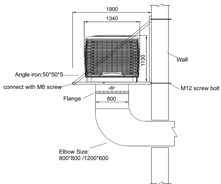
Foto 13 — Installazione del raffrescatore – Vista laterale
