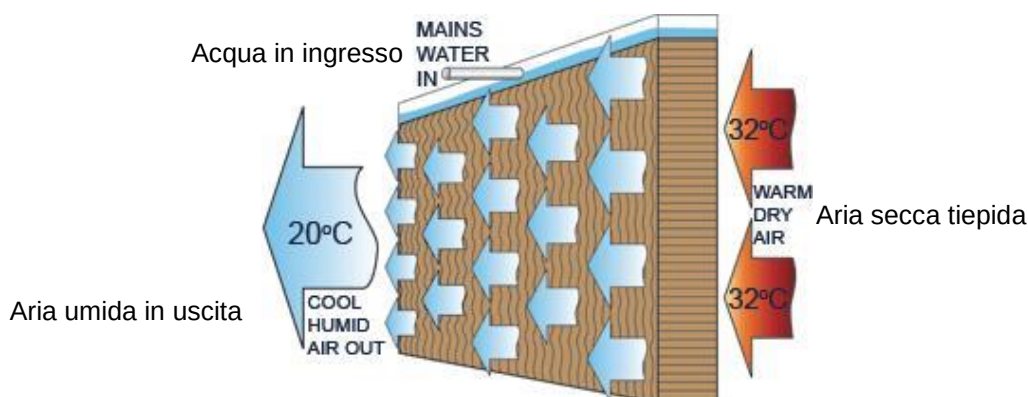
Figura 22 — Schematizzazione del processo di raffrescamento evaporativo
