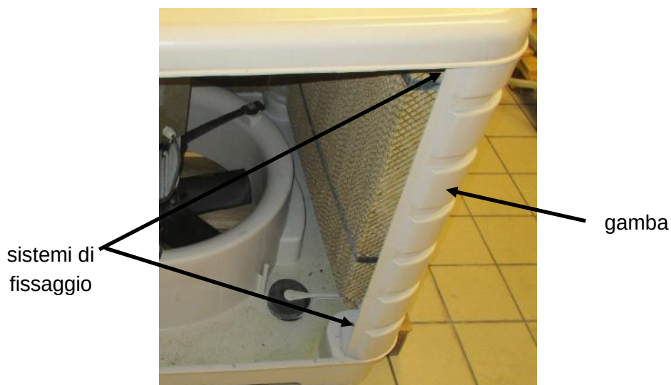
Foto 16 — Fissaggio della gamba alla struttura di base ed alla sommità della macchina
