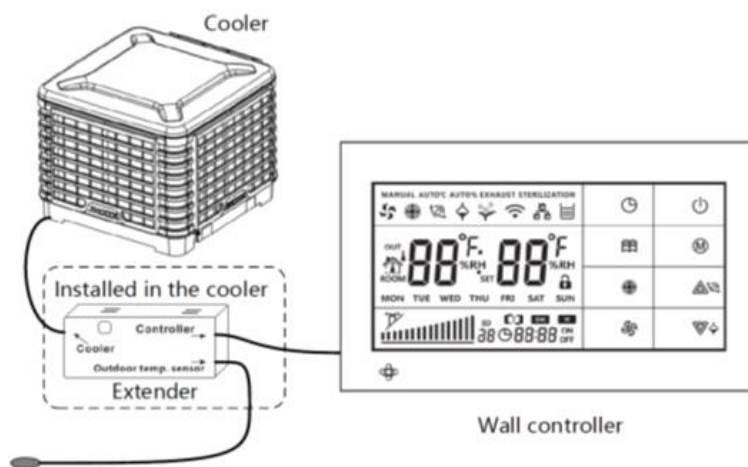
Figura 3 — Modalità di collegamento del quadro di controllo
