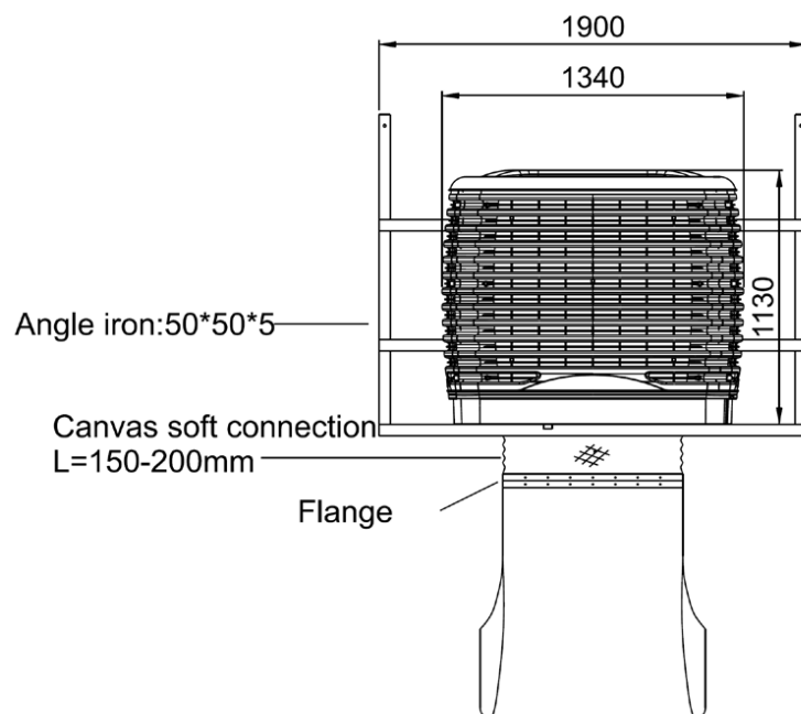
Foto 12 — Installazione del raffrescatore – Vista frontale
