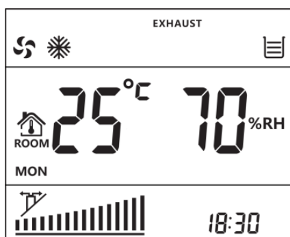
Figura 14 — Accensione della modalità scarico
