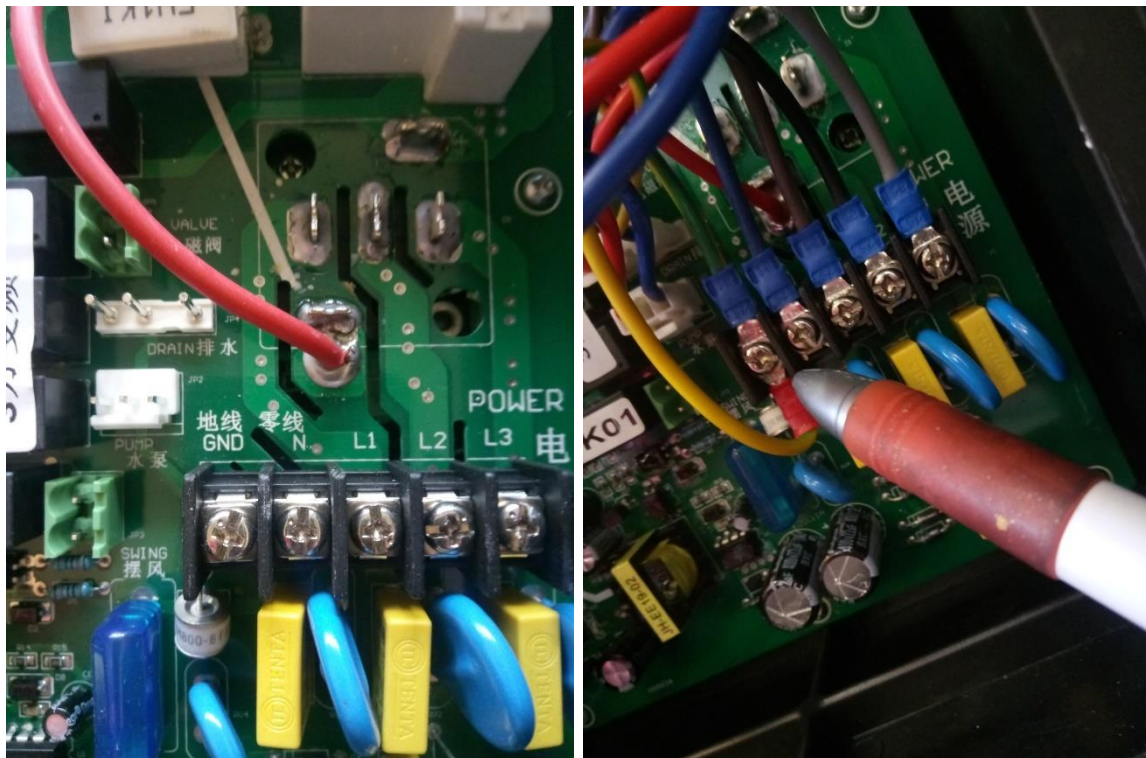
Foto 17 — Morsetti di collegamento dell'alimentazione elettrica e collegamento al circuito di protezione equipotenziale
