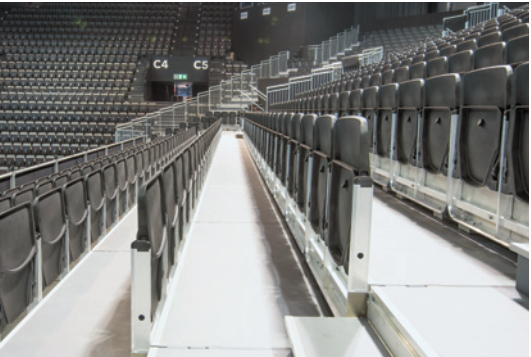
Bequeme Durchgangsbreite zwischen den Reihen von 72 cm.
