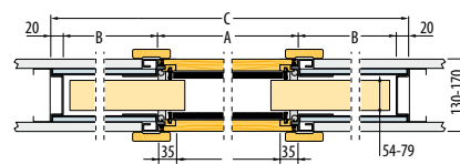
WYMIARY KASETY STANDARDOWEJ PODWÓJNEJ/ wersja do ściany murowanej i gips - karton
