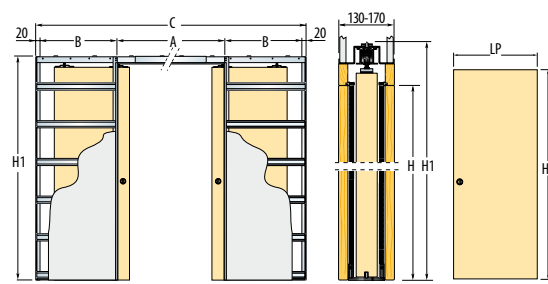
System przesuwny wewnętrzny podwójny
