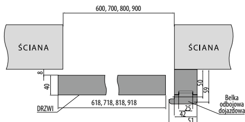
Rysunek systemu przesuwego naściennego bez zabudowy
