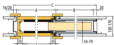
WYMIARY KASETY STANDARDOWEJ POJEDYNCZEJ/ do ściany murowanej i gips - karton
