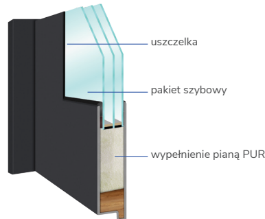
Przekrój skrzydła z pakietem szybowym
