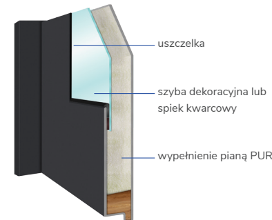
Przekrój skrzydła z aplikacją jednostronną
