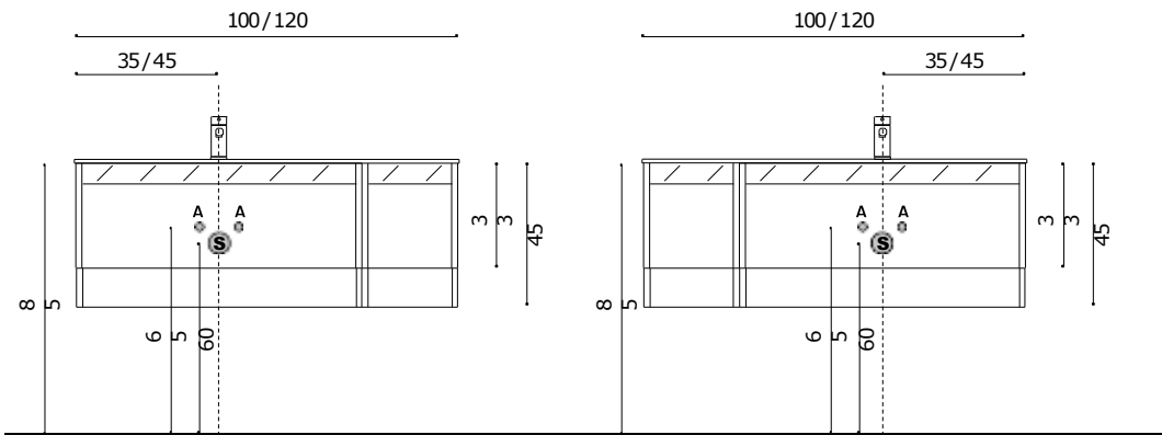
QUOTE BASI PORTALAVABO DECENTRATE CON MODULO DA 30 L.100 (70+30)/L.120 (90+30) LAVABO H.1,3 QUOTAS DISCHARGES DECENTRALIZED BASE UNIT FOR WASHBASIN H. 1.3 W.100 (70+30)/W.120 (90+30)
