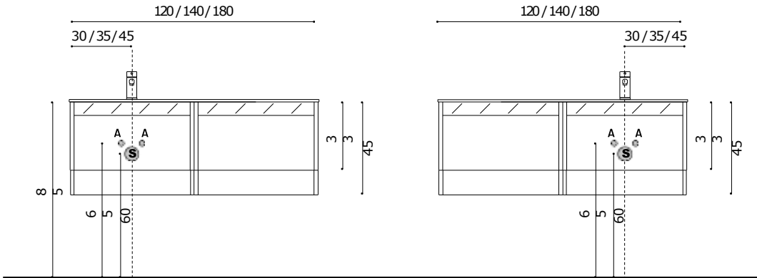
QUOTE BASI PORTALAVABO DECENTRATE CON LAVABO H.1,3 QUOTAS DISCHARGES DECENTRALIZED BASE UNIT FOR WASHBASIN H.1,3
