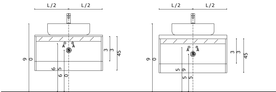
QUOTE BASI PORTALAVABO PER TOP CHIUSURA H.2 E TOP SCATOLARE H.5 QUOTAS DISCHARGES FOR CLOSING TOP H.2 AND BOX-SHAPED TOP H.5
