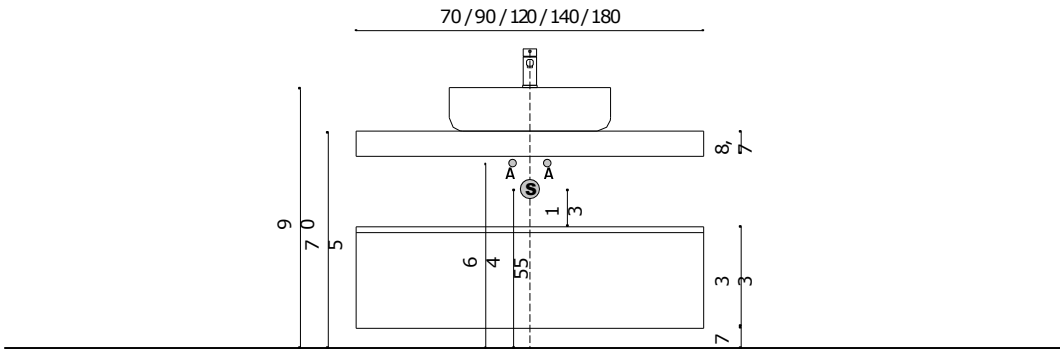
QUOTE PER TOP SCATOLARI CON BASI H.33 QUOTAS DISCHARGES FOR BOX-SHAPED TOP WITH BASE UNIT H.33
