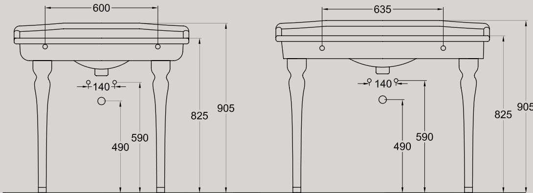
Gamba D35 per consolle D31 Leg D35 for D31
