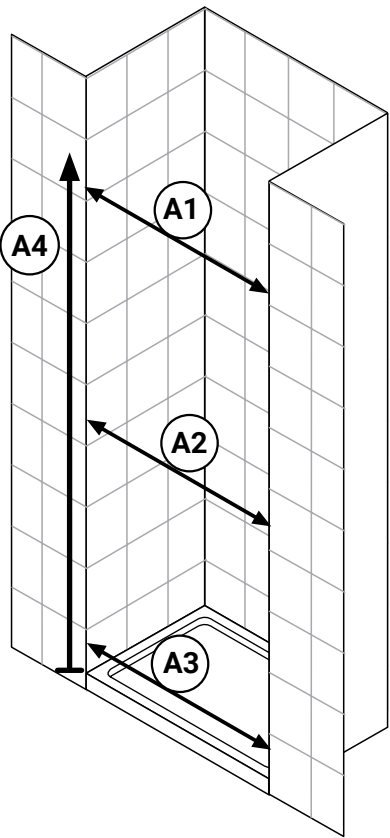
"C" - Spazio in nicchia semi incassata Dx Semi-recessed niche right - Halbversenkte Nische rechts Niche semi-encastée à droite
