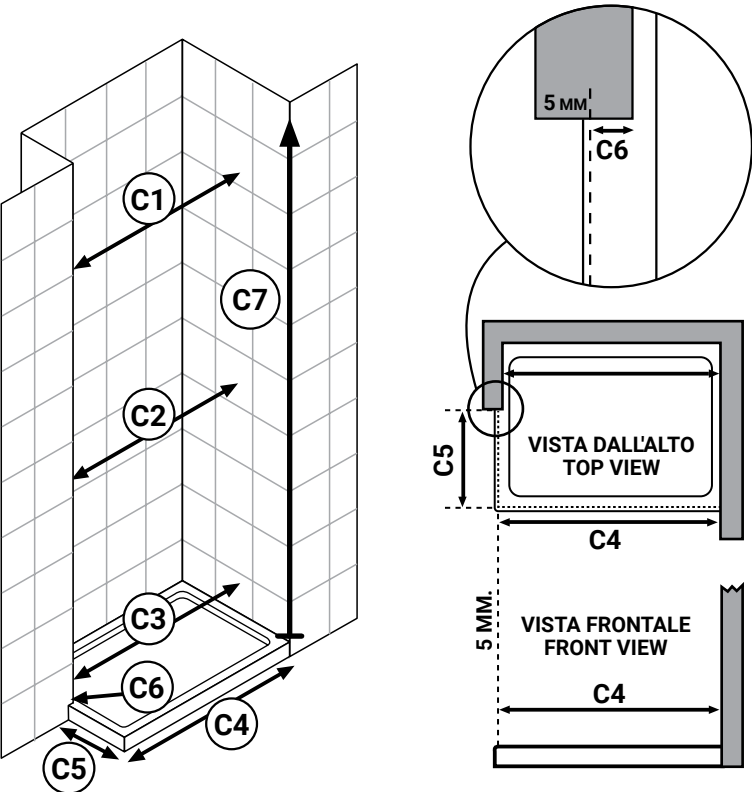
"C" - Spazio in nicchia semi incassata Dx Semi-recessed niche right - Halbversenkte Nische rechts Niche semi-encastée à droite
