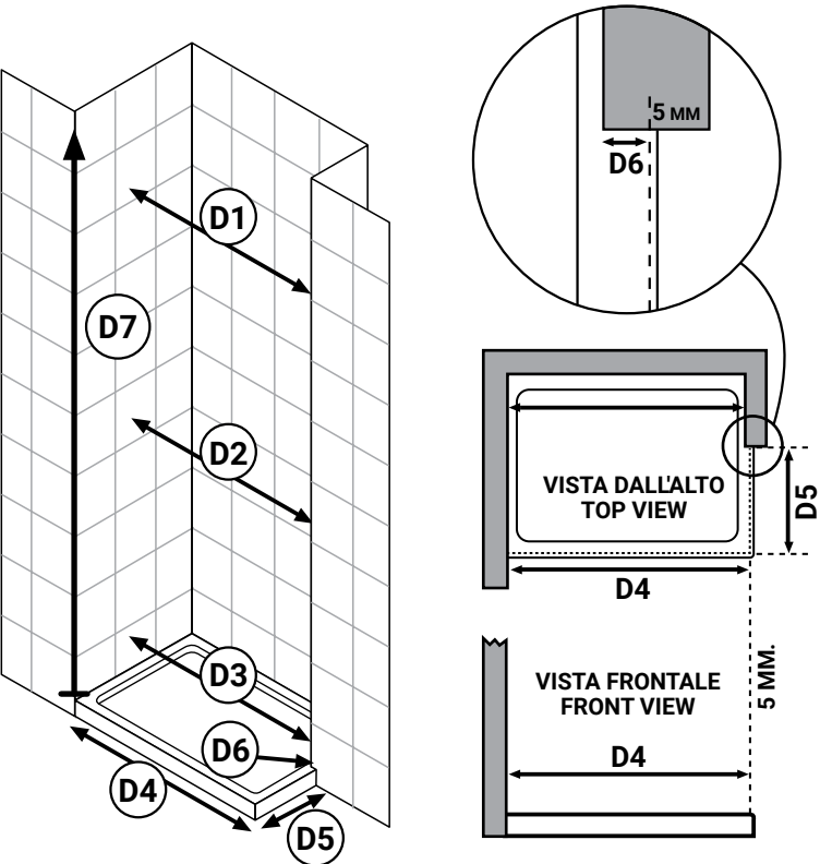
"D" - Spazio in nicchia semi incassata Sx Semi-recessed niche left - Halbversenkte Nische links Niche semi-encastée à gauche
