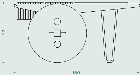
VISTA SUPERIOR TOP VIEW VISTA DALL'ALTO
