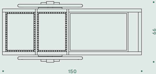
VISTA SUPERIOR TOP VIEW VISTA DALL'ALTO
