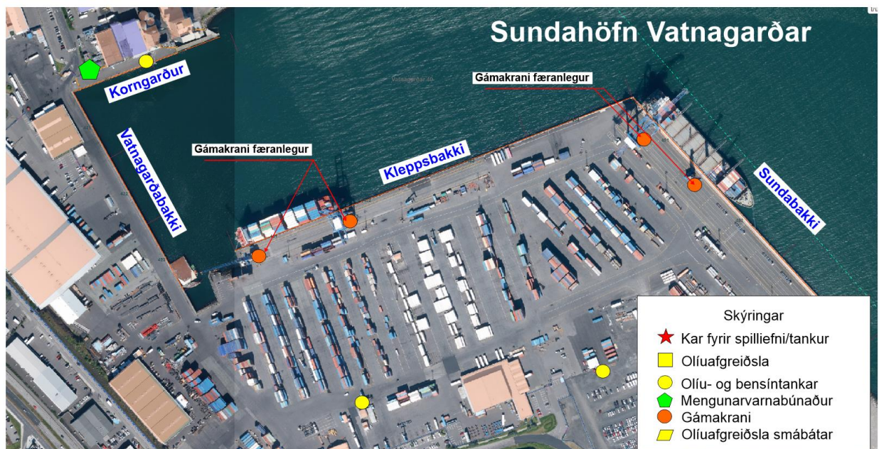
Mynd 5: Reykjavík – Sundahöfn: Vatnagarðar; Korngarður, Sundabakki, Kleppsakki.
