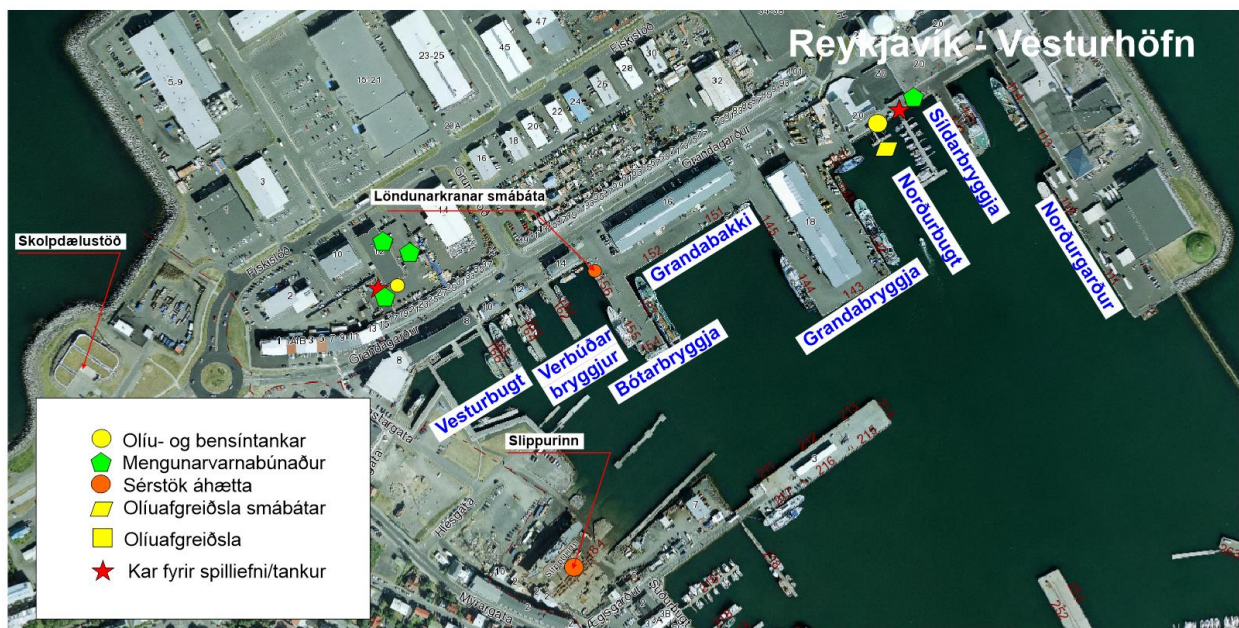
Mynd 2: Reykjavík - Gamla höfnin: Vesturhöfn; Norðurgarður, Síldarbryggja, Norðurbugt, Grandabryggja, Grandabakki, Bótarbryggja, Verðbúðarbryggjur, Vesturbugt.
