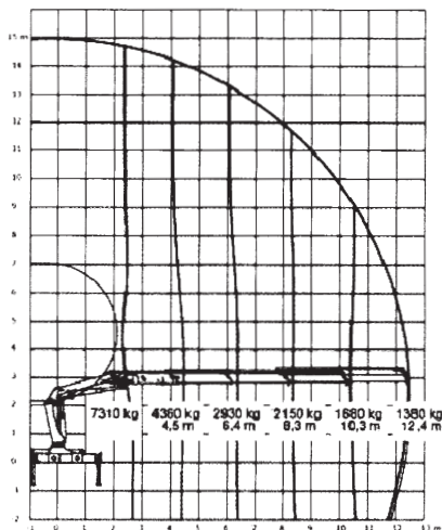
Belastungsdiagr. HMF 2200-K4
