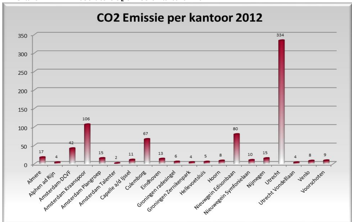
Grafiek 4: Absolute CO 2 emissie kantoren 2012
