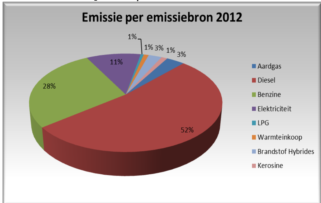
Grafiek 6: Absolute CO 2 emissies per emissiebron - 2012
