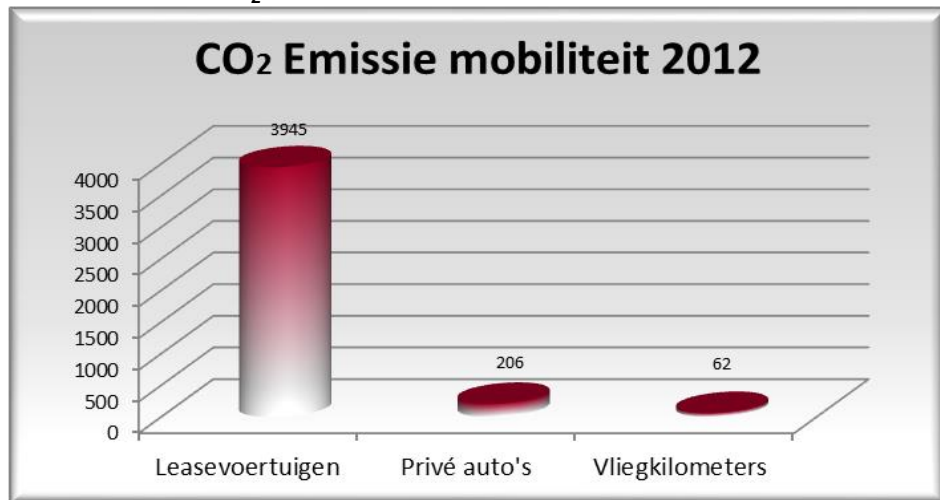
Grafiek 3: Absolute CO 2 emissie mobiliteit 2012
