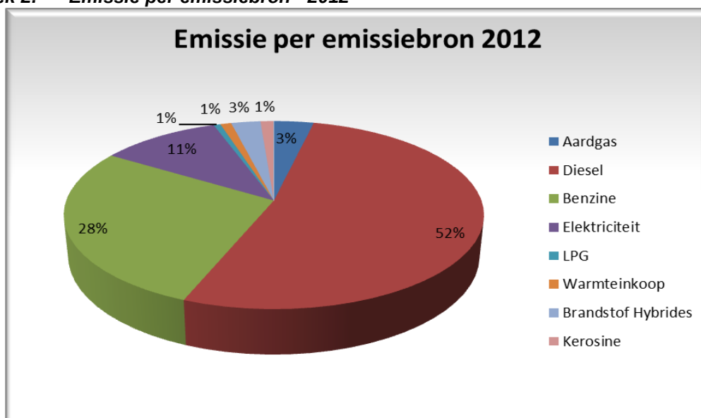
Grafiek 2: Emissie per emissiebron - 2012
