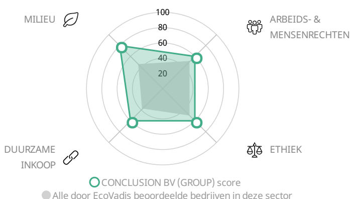
Vergelijking thema-score
