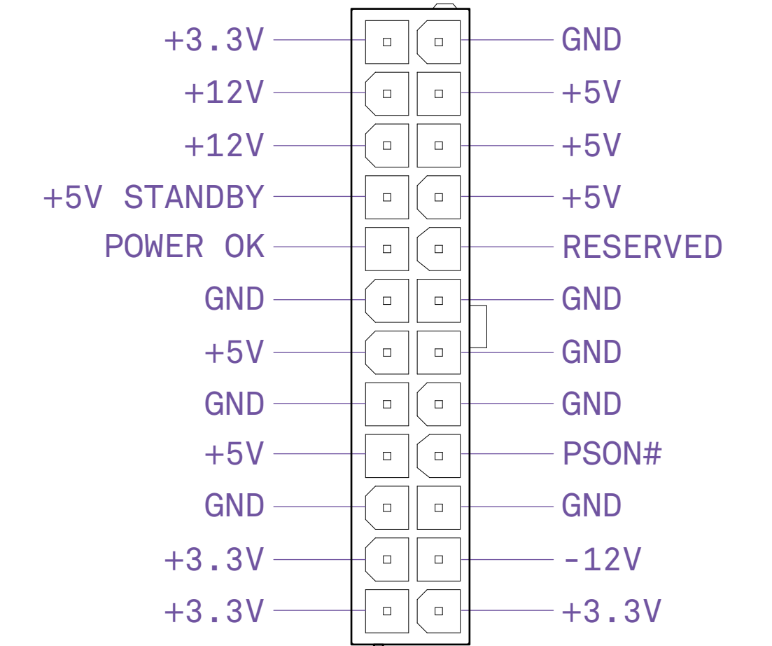
ATX_PWR
