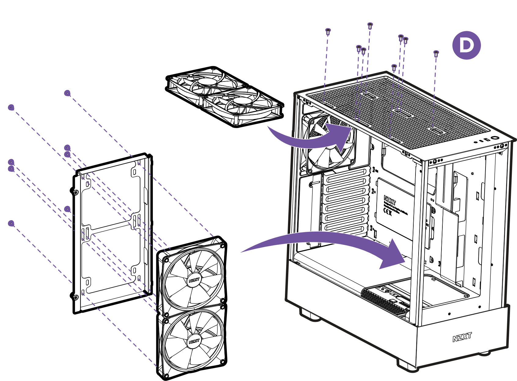
ВЕНТИЛЯТОРА
