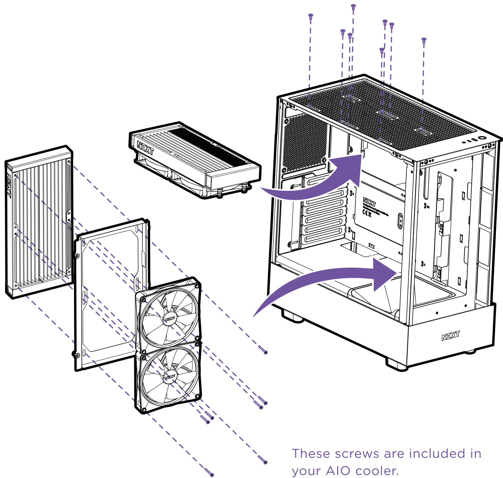
RADIADOR
