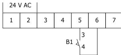
Morsettiera circuiti ausiliari X1
