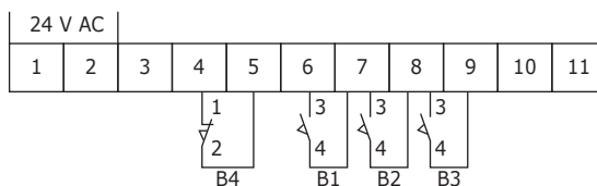
Morsettiera circuiti ausiliari X1
