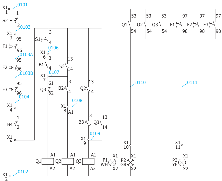
Morsettiera circuiti ausiliari X1
