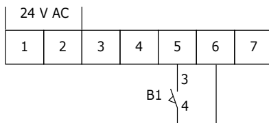
Morsettiera circuiti ausiliari X1
