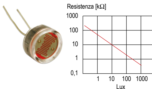
Fotoresistore e caratteristica elettrica.
