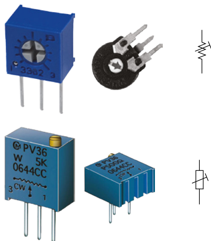
Trimmer, trimmer multi giro e relativi simboli elettrici.
