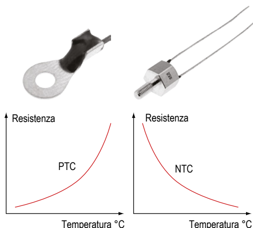
Termistori e caratteristica elettrica.
