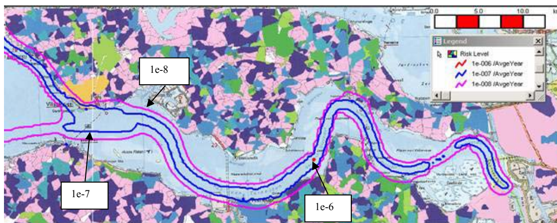
Figure 8.3 – Basis Case Ontvlambare Gassen Plaatsgebonden Risico Contouren
