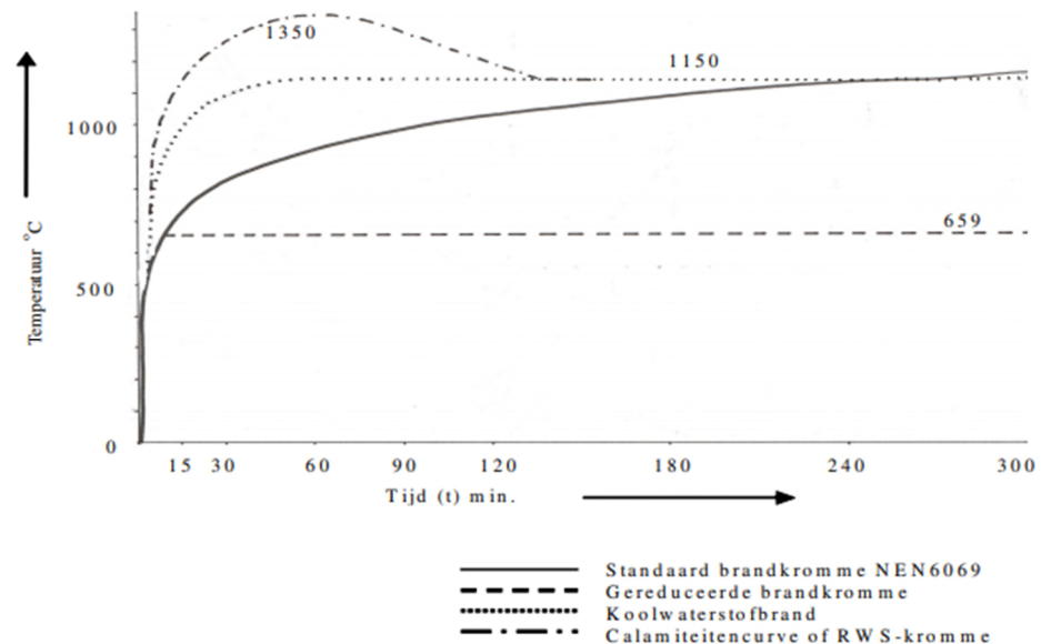
Fig. 1.1: nominale brandkrommen (temperatuur-tijd krommen)
