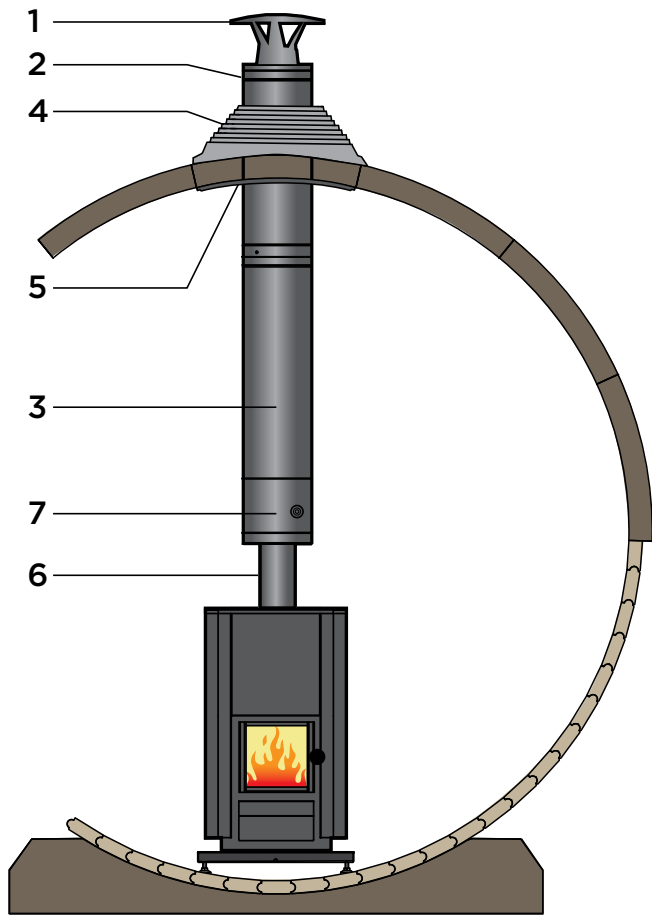
Tünnisauna korstna näidis
