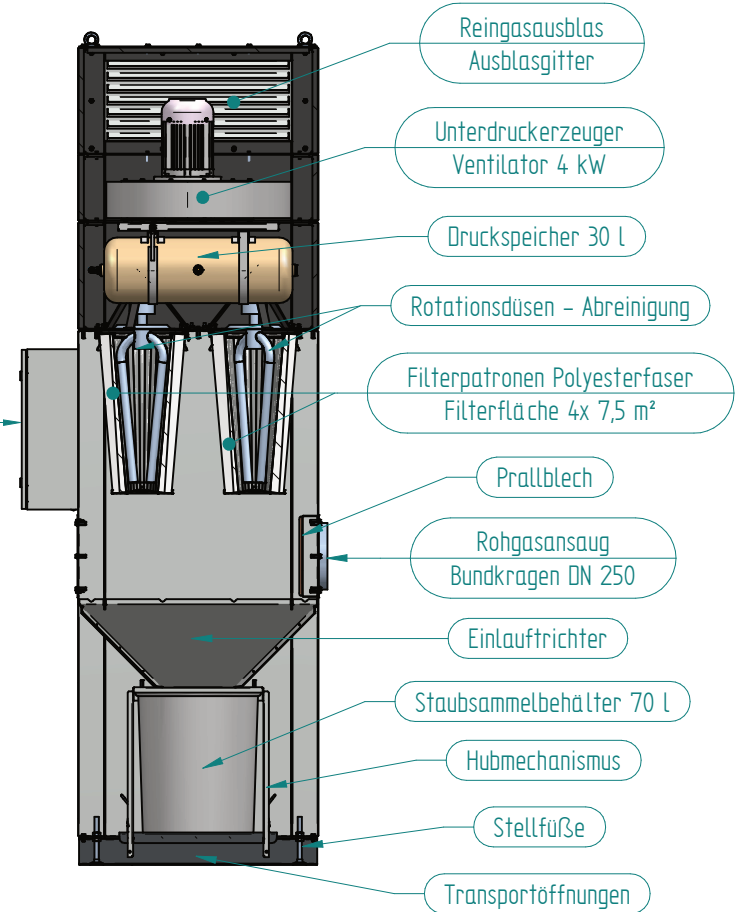
Schnitt A-A
