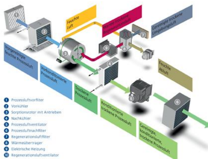
Abb. 5: Funktionsschema der Sorptions-Lufttrocknung
