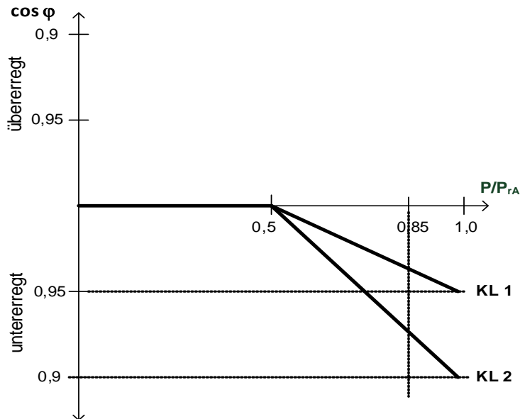
Bild 1 \cos \phi = f(P/P_{rA}) Standardkennlinien für EZA mit P_{rA} < 135 \text{ kW} Erläuterung: EZA Typ 1 = direkt gekoppelte Synchrongeneratoren EZA Typ 2 = Anschluss über Wechselrichter (PVA), direkt gekoppelte Asynchronmotoren (ASM)
