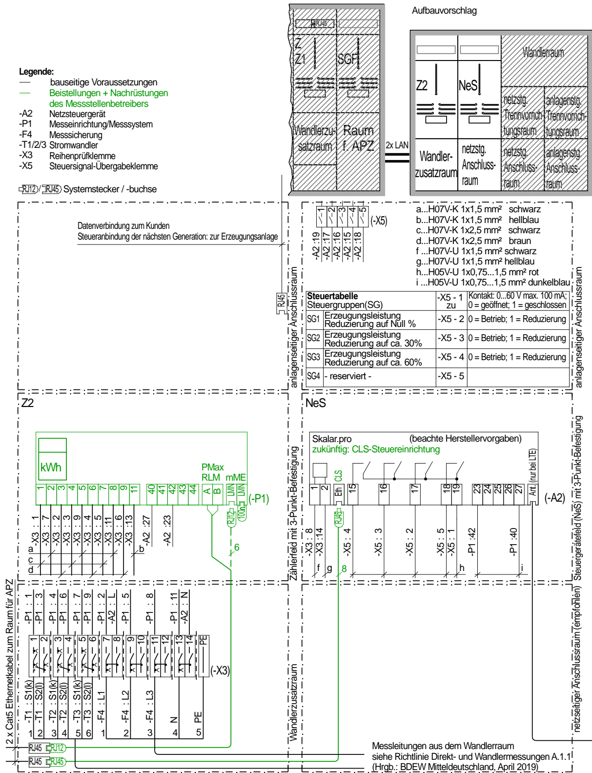
Bild 2 Aufbau Zählerplatz / NeS-Platz Anlagenklasse 1 (Wandlerrmessung)
