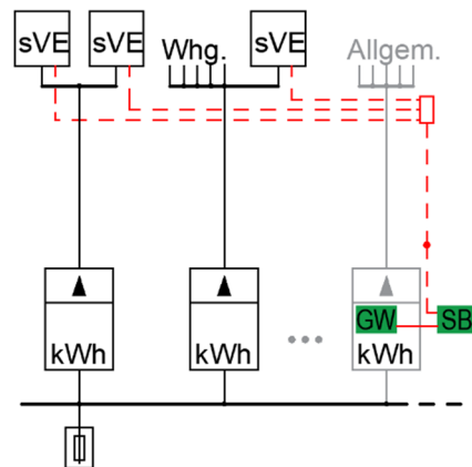
Bild 6: Prinzip direkte Steuerung als Gruppe
