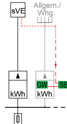
Bild 4: an Mehrkundenanlage oder EFH mit 2 Zählern
