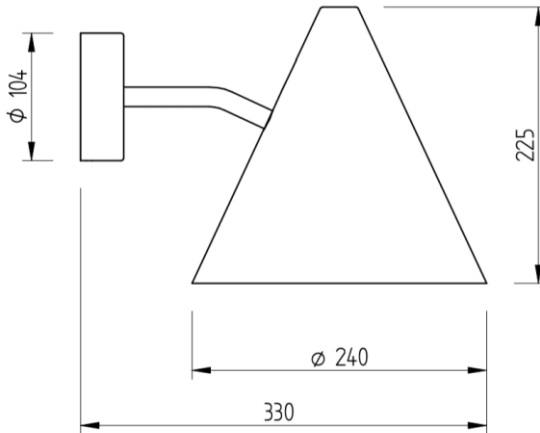
Fig 3. Armaturens yttermått / The luminaire dimensions
