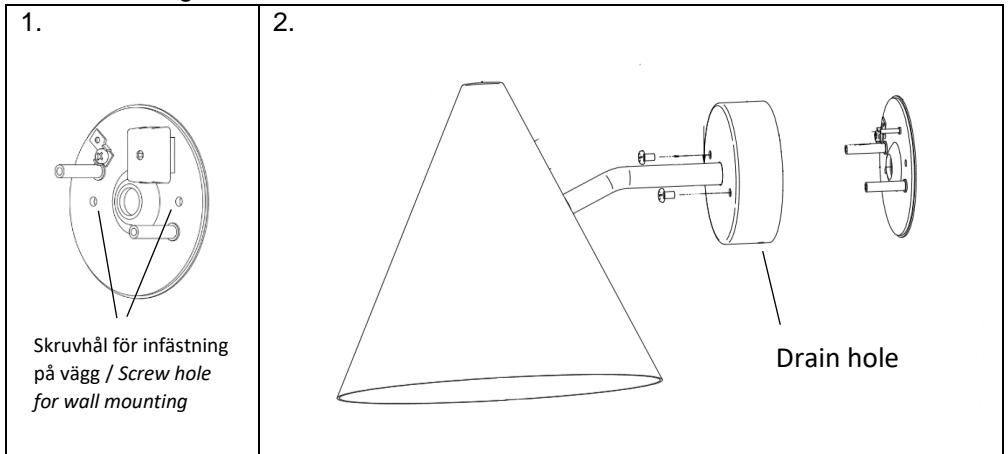
Fig 2 1. Väggfäste / 1. Wall bracket. 2. Monteringsanvisning för montering på vägg med markerat dränagehål. / 2. Mounting instruction for mounting on a wall with marked drain hole.
