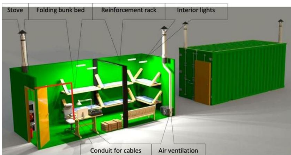
Обустройство блиндажа
