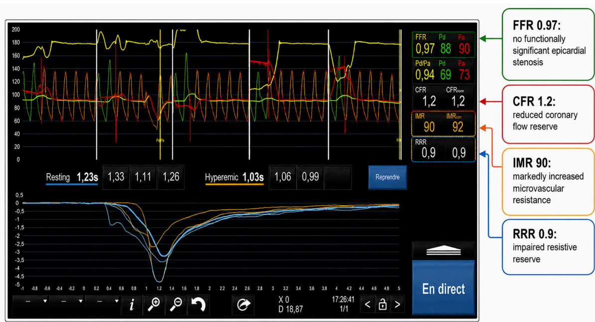
Figure 2 : Test invasif de la microcirculation coronaire positif, associant l'absence de sténose épicaudique fonctionnellement significative (FFR 0,97) à une réserve coronaire diminuée (CFR 1,2), une résistance microvasculaire élevée (IMR 90).
