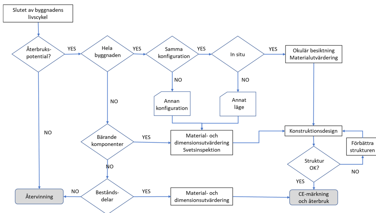
Figur 12: Schematisk process för att välja hur man ska hantera stål återbruk i samband med att en byggnad nått slutet på sin livscykel. Fritt översatt från Coelho et al. (2020).
