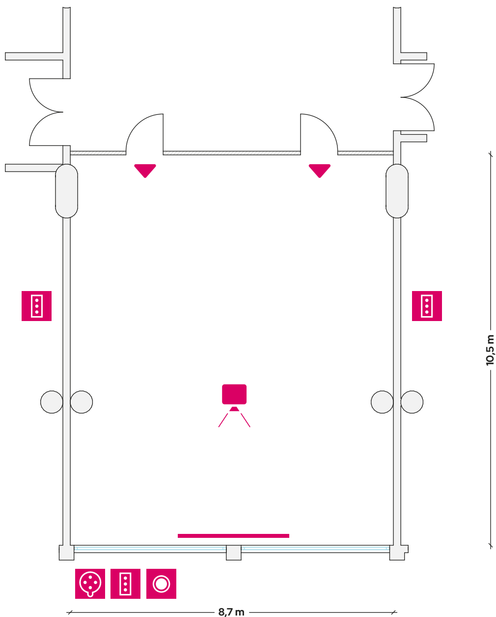
Pianta rapp. 1:100
