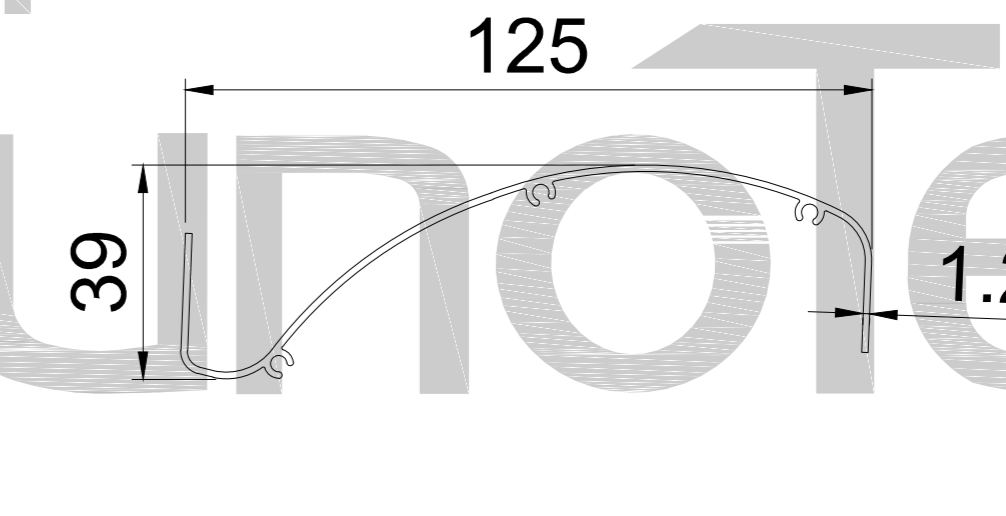
Louver Blade
