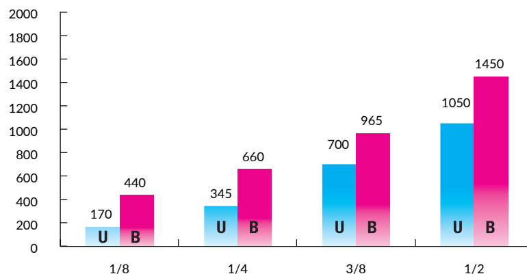
Portata - Flow capacity - Débit - Durchflusswerte [l/min] 6 bar - Δp1
