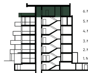
ŘEZ DOMU
