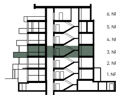
ŘEZ DOMU
