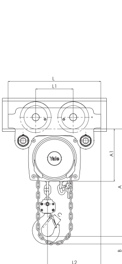
Yalelift ITG, 500 - 3000 kg, single fall
